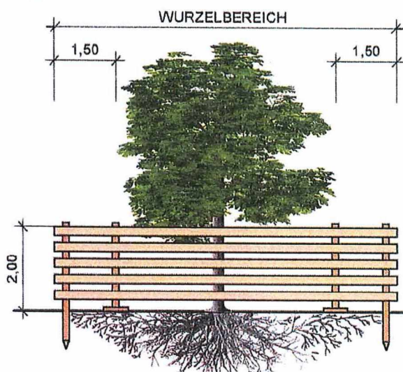
Variante A WURZELSCHUTZ DURCH ZAUN
